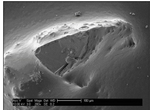
P60g Zirconia - SEM
